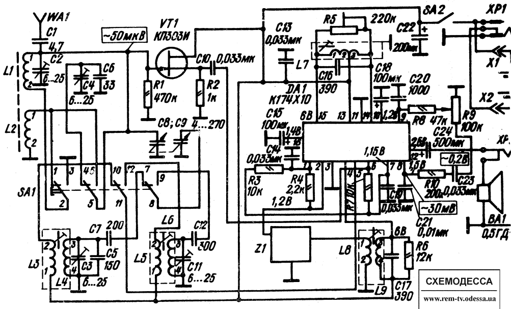
Принципиальная электрическая схема приемника "ВЕГА-341" (переключатель диапазона в положение ДВ)
