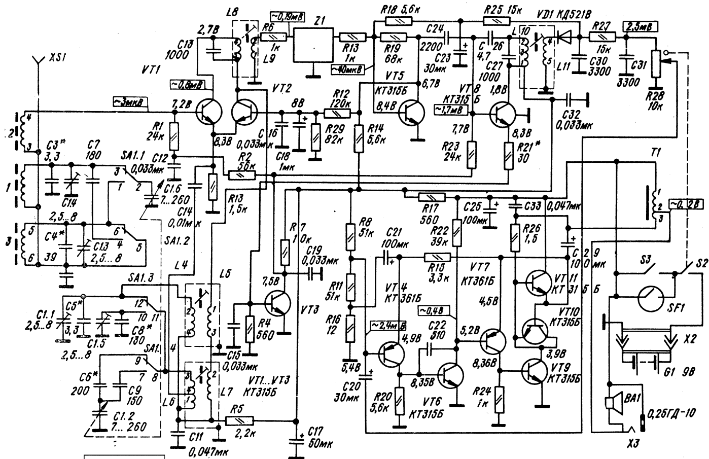
Принципиальная электрическая схема приемника "СИГНАЛ-304" (переключатель диапазонов в положении СВ)
