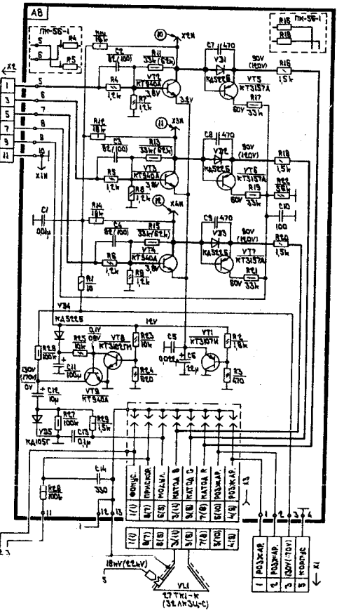
Плата кинескопа ПК-56 (ПК-56-1)
